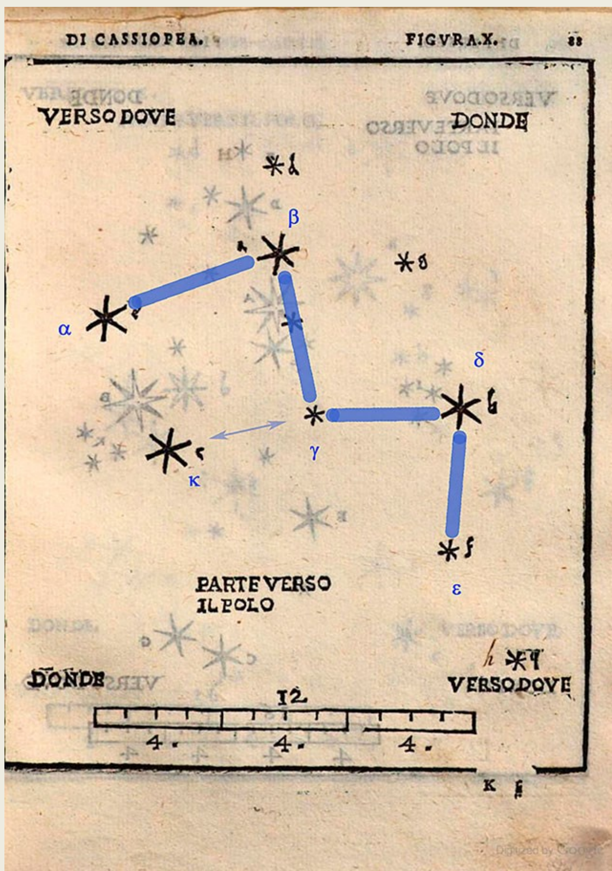
[Илл. 06-22-02-1. Allesandro Piccilomini, Атлас звёздного неба «De la Sfera del Mondo. Dele Stelle fisse», Venetia, 1540, f.88, Figura X.]
