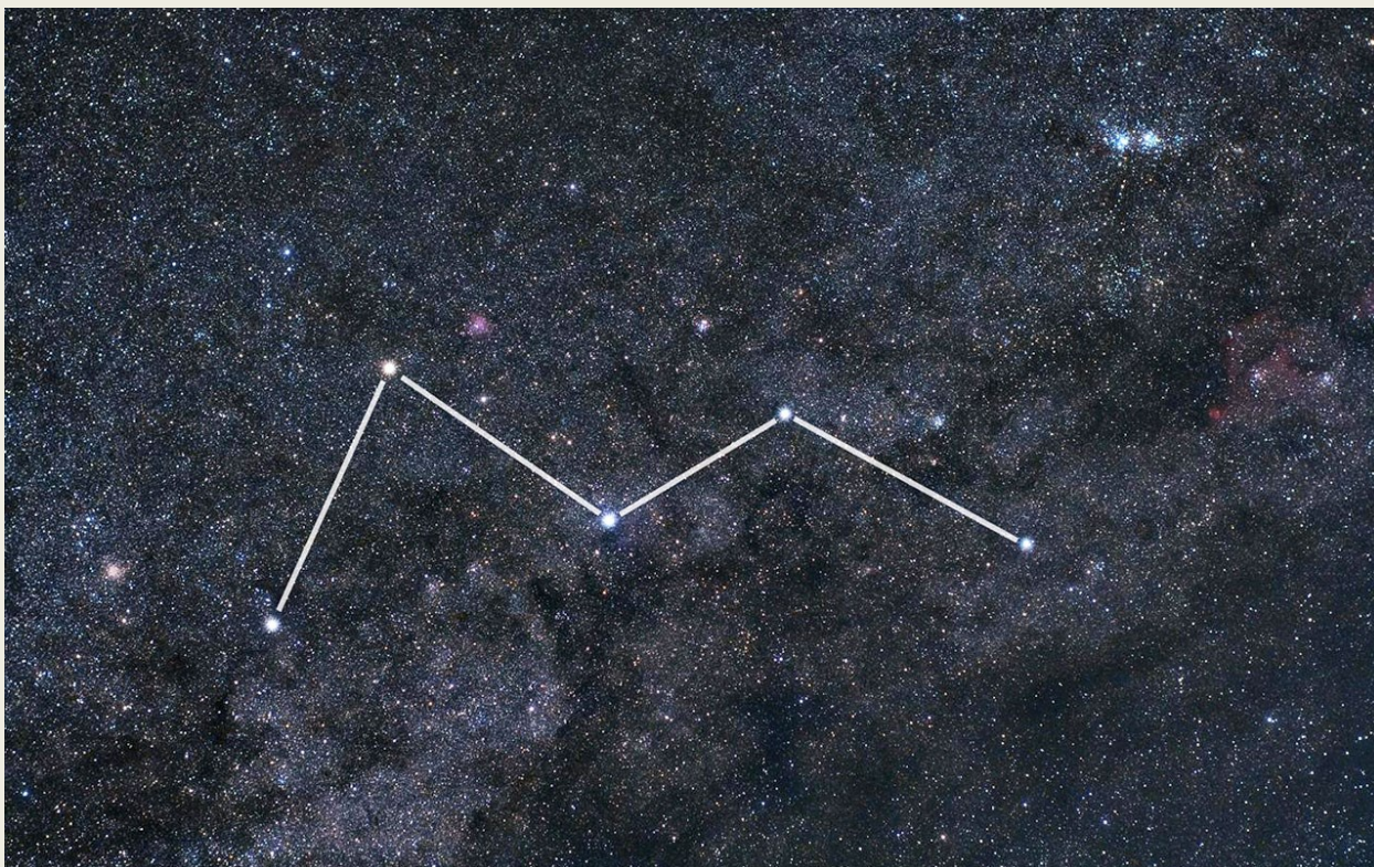
[Илл. 06-22-01-1. Созвездие Кассиопеи.]
